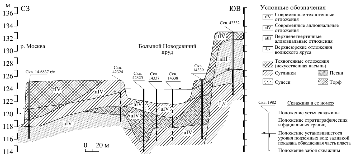
Рис. 2. Схематический геолог-литологический разрез по линии, перпендикулярно пересекающей Большой Новодевичий пруд в его северо-восточной части (по данным ЗАО
