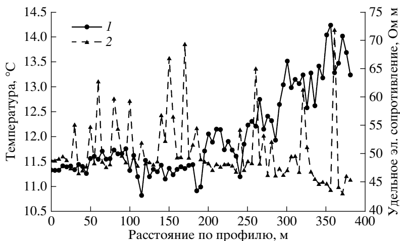
Рис. 9. Графики температуры и удельного электрического сопротивления воды на урезе вдоль берега Большого Нововедвичьего пруда. Условные обозначения: 1 – температура на урезе воды; 2 – удельное электрическое сопротивление на урезе воды.
