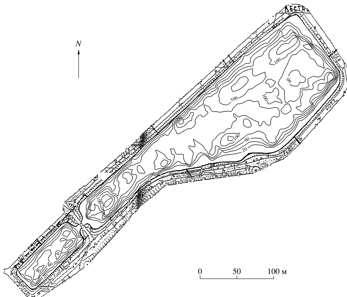
Рис. 6. Карта изопакит современных осадков (верхнего комплекса) Большого и Малого Новодевичьих прудов. Сечение изолиний 20 см.
