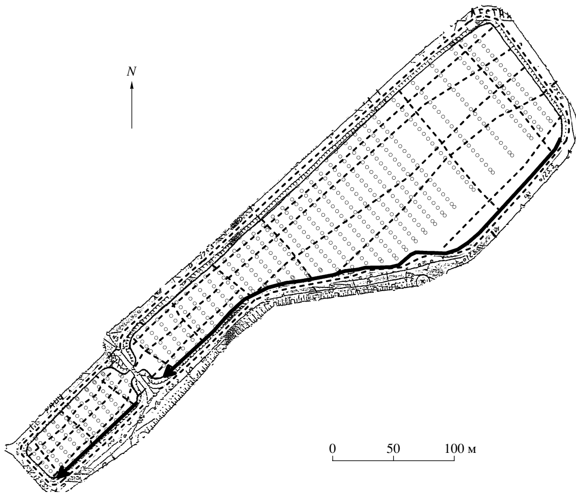
Рис. 1. Карта фактического материала в районе исследования. Условные обозначения: пунктирные линии – радиолокационные профили; пустые кружки – точки измерения потенциала ЕП; жирные линии – профили термометрии и резистивиметрии (начало профиля обозначено стрелкой).
