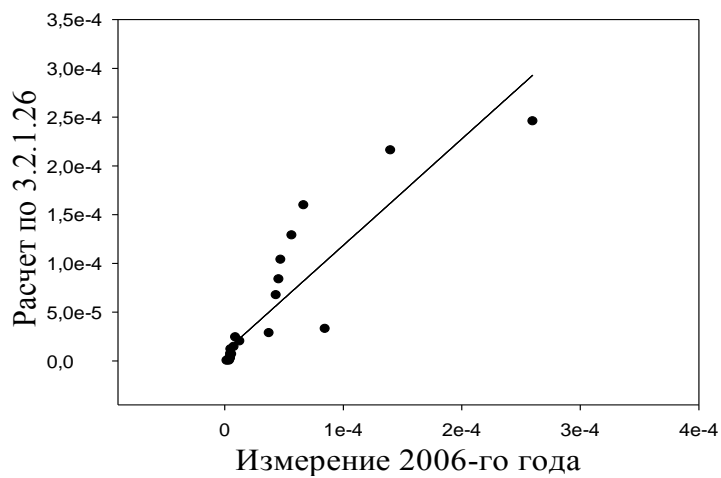
Рис. 1. Проверка соответствия результатов прогноза по модели (26) аналитическим измерениям 2006 г.
