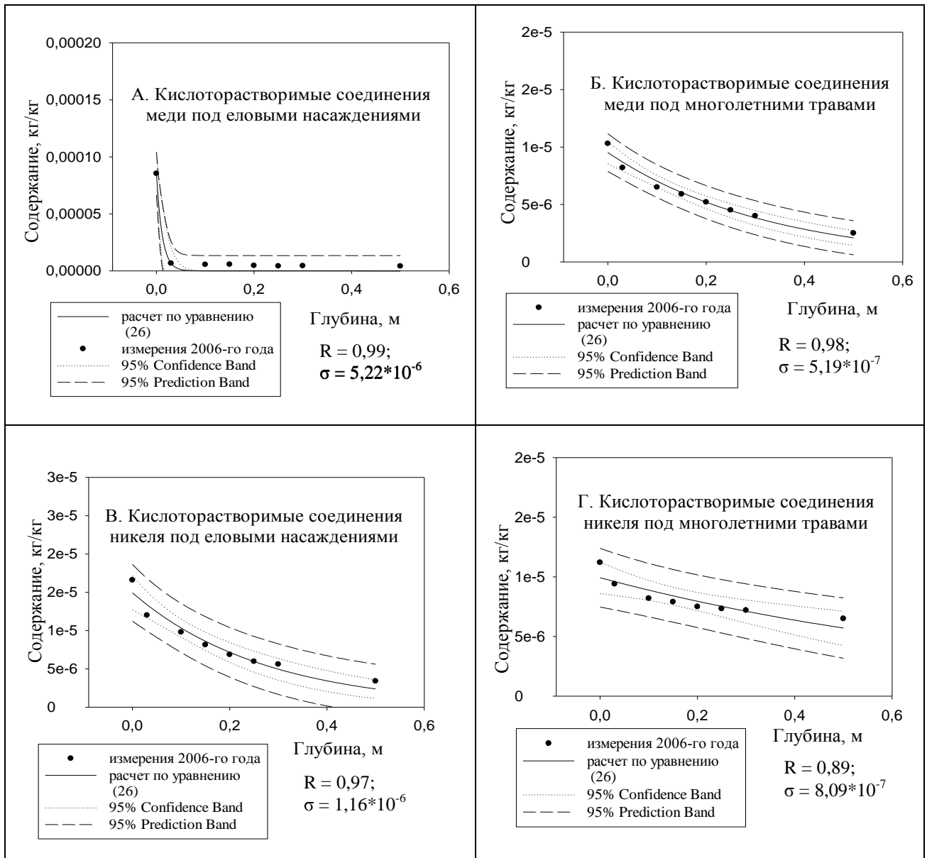
Рис. 2. Прогнозирование содержания ТМ в почве лизиметров под различными видами растительности (точки – опыт, линии – модель (26) и доверительные пояса для средних (Confidence band) и для прогнозных величин (Prediction band) при P=95\% )
