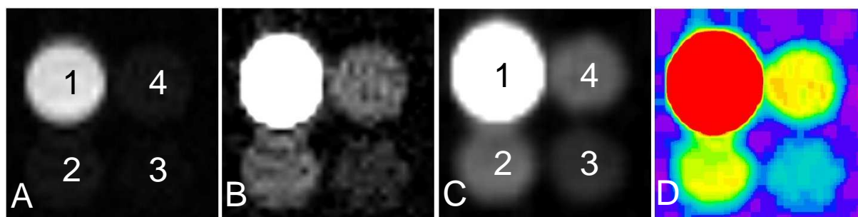
Рис. 7. МРТ изображения перфтордекалина (1) и эмульсии, содержащей перфторан (2-4) при разных вариантах графической обработки. TR/TE=300/5.1 мс, FOV= 64x64мм, N=32, (10 мин).
