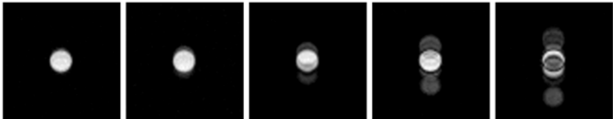
Рис. 6. МР-изображения флакона с перфтордекалином при разных значениях BW (в кГц) - слева направо: 41.6, 20.8, 11.6, 6.5, 4.4. FOV=128 \times 128 мм, N=64 .
