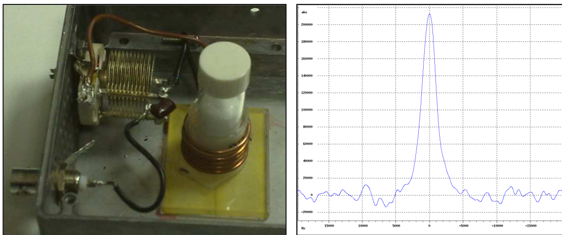
Рис. 1. Слева – датчик для регистрации ЯКР. Справа – спектр ЯКР ^{35}\text{Cl} от \text{KClO}_3 ( \text{SW}=40 кГц, \tau=40 мкс, \text{NS}=1 ).
