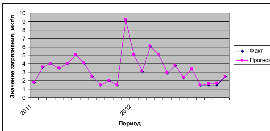
Рис. 1. Сопоставление фактического и прогнозного значений уровня загрязнения нитритами вод в районе МГ «Ялта» при использовании метода Винтерса
