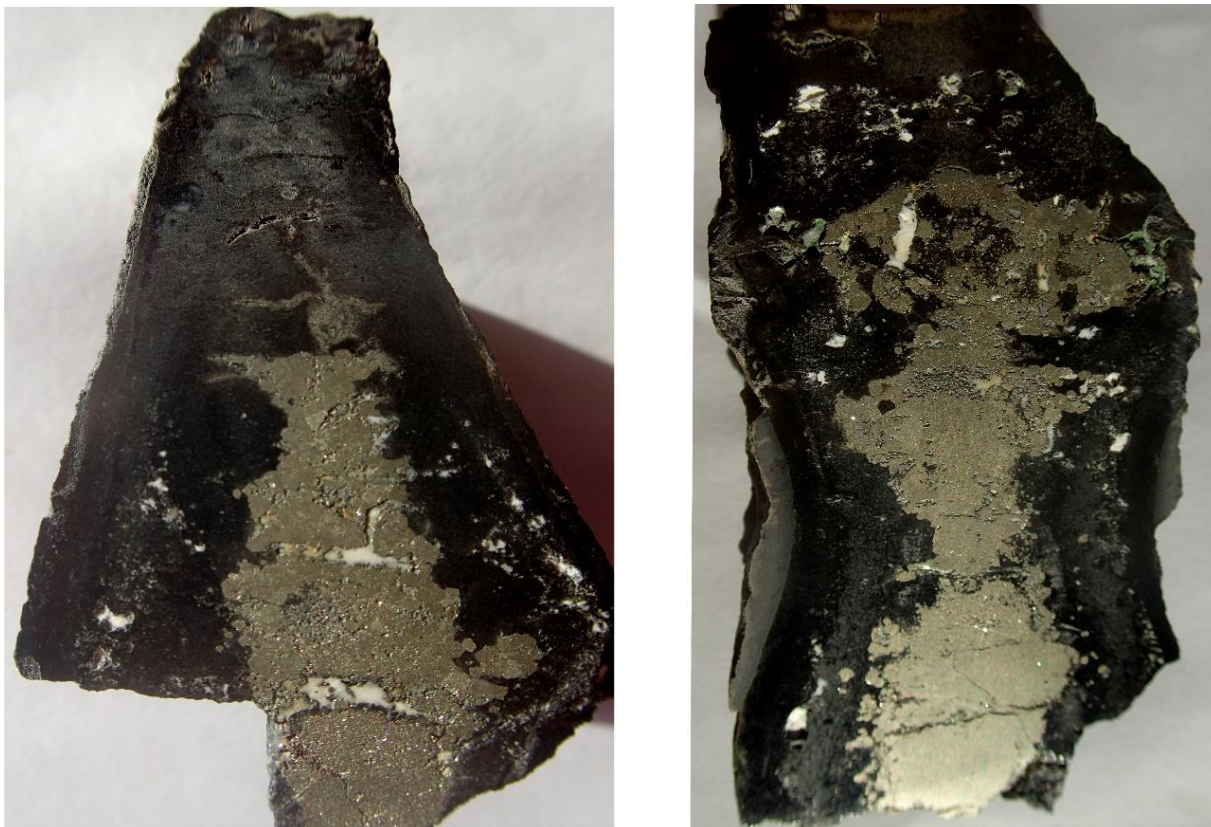
Рис. 2. Зональное строение сульфидно-карбонатных построек с флюидным каналом в центральной части
