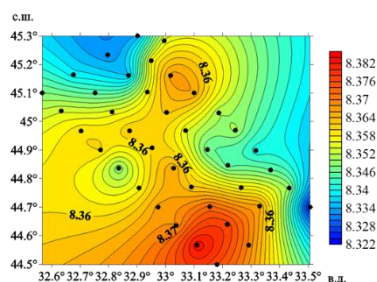
Рис.1. Распределение величины рН на поверхности 7-10 июня 2016 г.
