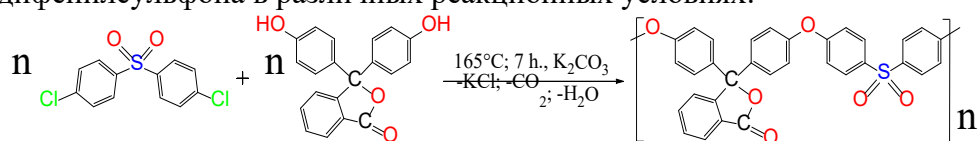
Рисунок № 1. Синтез полисульфона
