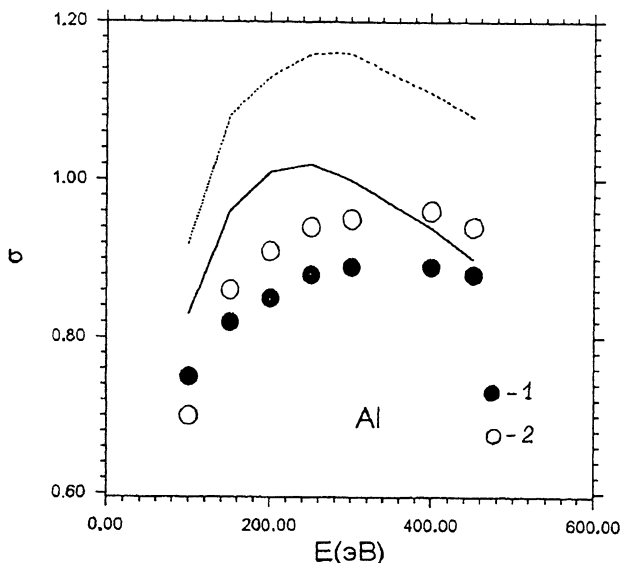
Рис. 1. Общий выход электронов в зависимости от энергии электронного пучка. Расчетные значения, полученные для газа не- и взаимодействующих электронов: штриховая и сплошная линии соответственно. Эксперимент: 1 — [13], 2 — [14].
