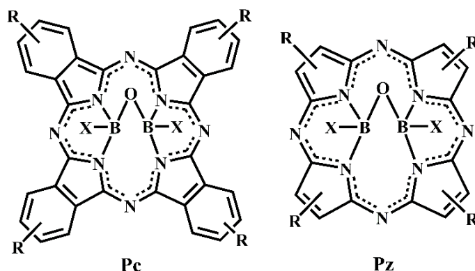
Рисунок 1. Структура замещенных диборных комплексов фталоцианина (Pc) и порфираина (Pz).
