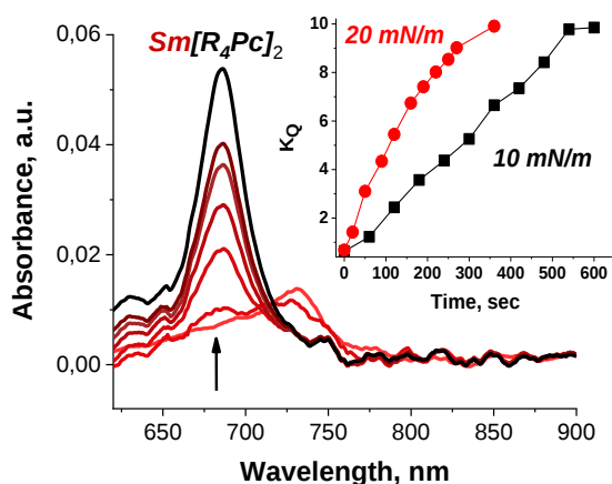
Рис. 1 Эволюция спектров поглощения монослоя \text{Sm}[(15\text{C}5)_4\text{Pc}]_2 при 10 мН/м на поверхности раздела воздух/вода при УФ-облучении. На вставке показаны кинетические кривые УФ-индуцированной редокс-изомеризации при 10 (черная кривая) и при 20 (красная кривая) мН/м.
