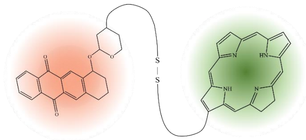
Рисунок 1. Общая структура полученных соединений
