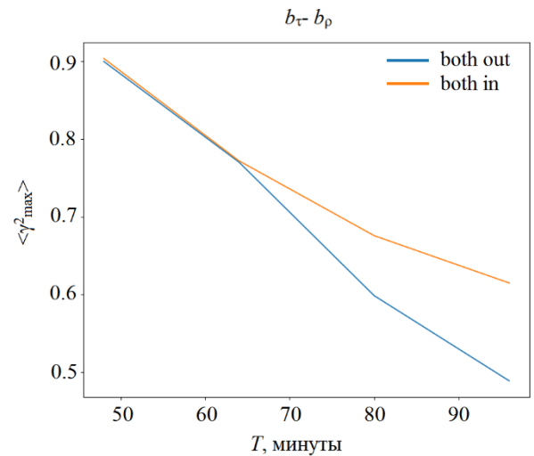
Рис. 2. То же для пары компонент b_z - b_p
