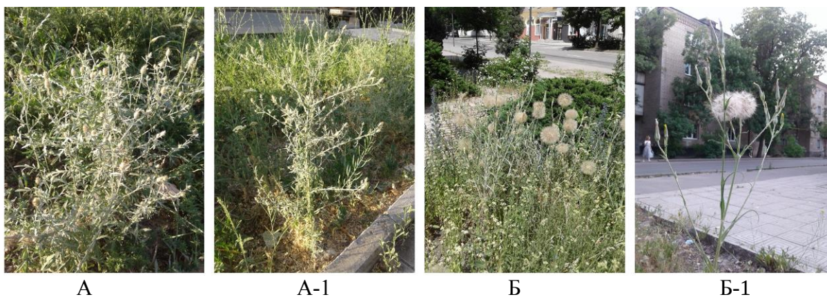
Рис. Габитуальная контрастность астровых при полицентрическом (А, Б) и моноцентрическом (А-1, Б-1) побегообразовании.
