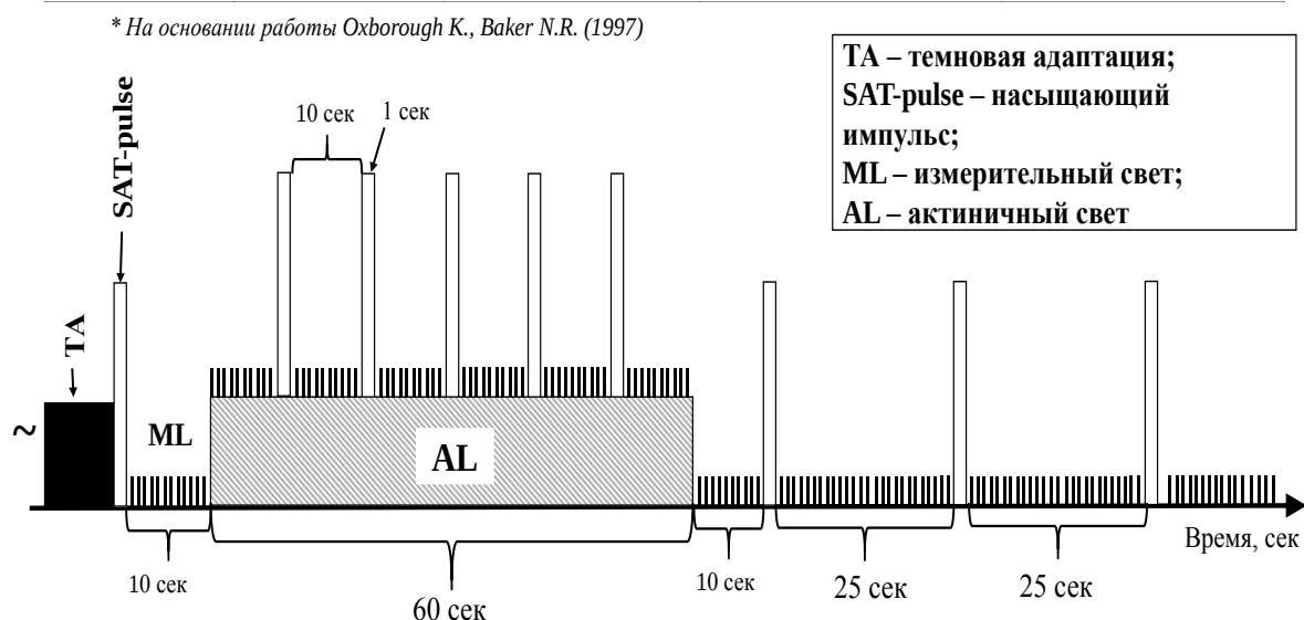
Рис. 1. Протокол измерения показателей нефотохимического тушения флуоресценции
