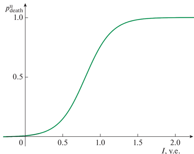
Рис. 4. Зависимость вероятности гибели клетки p_{\text{death}}^u от уровня освещенности при N_{\text{cells}}^u = 2000 , q_i^u = 35 . Расчетная формула приведена в табл. 1.
