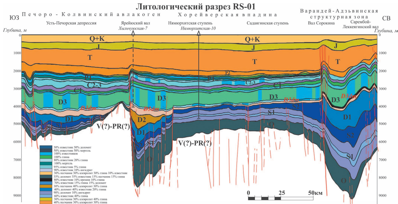
Рис. 8. Литологическая модель разреза RS-01 (длина 270 км, глубина 9,3 км)
