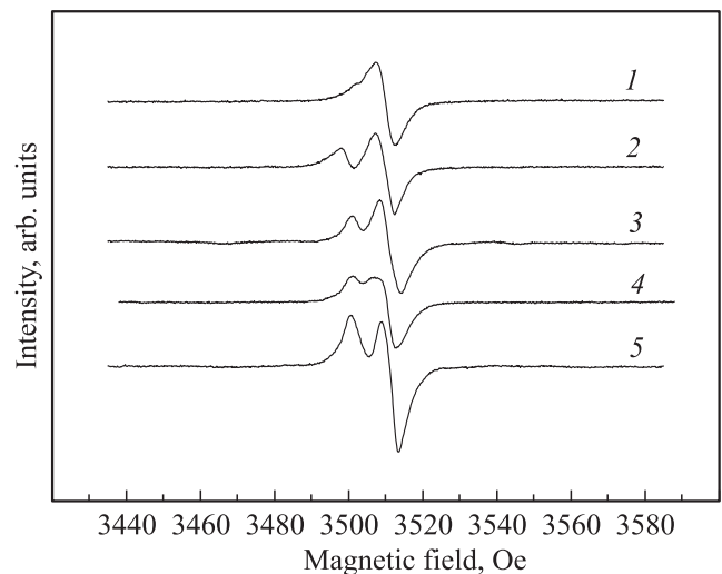
Рис. 4. ЭПР спектры поглощения СВЧ излучения: 1 — до напуска ПБХ, 2 — после напуска ПБХ, 3 — спустя 2 месяца, 4 — после воздействия на образец УФ-облучения, 5 — после извлечения образца на воздух.
