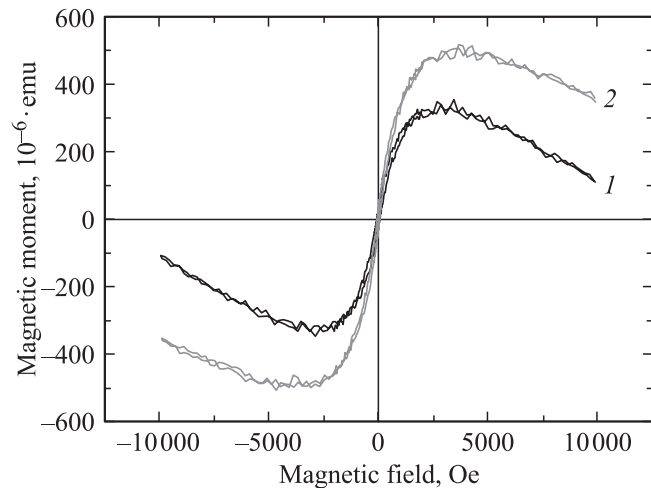
Рис. 2. Зависимость магнитного момента от величины магнитного поля для структур „образец + шток“ после напуска ПБХ: 1 — первый образец, 2 — второй образец.
