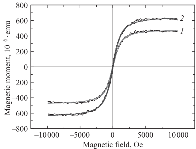
Рис. 3. Зависимость магнитного момента от величины магнитного поля (после учета диамагнитного вклада): 1 — первый образец, 2 — второй образец. Сплошные кривые — аппроксимация экспериментальных данных функциями Ланжевена.
