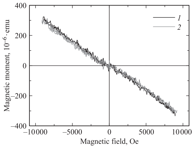
Рис. 1. Зависимость магнитного момента от величины магнитного поля для структур „образец + шток“ до напуска ПБХ: 1 — первый образец, 2 — второй образец.
