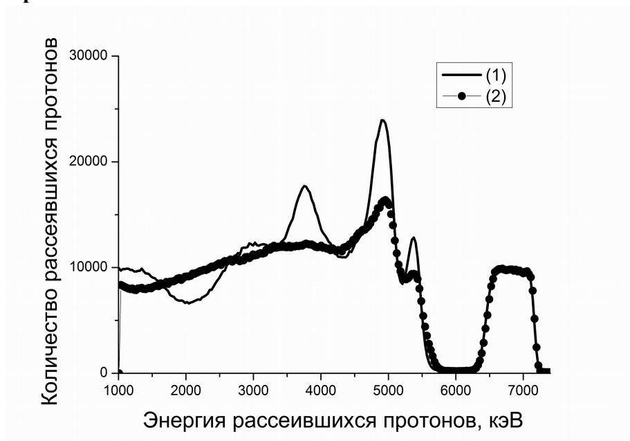
Рисунок. Сравнение спектров ЯОР от пластинки магния (1) и порошкообразного магния (2)
