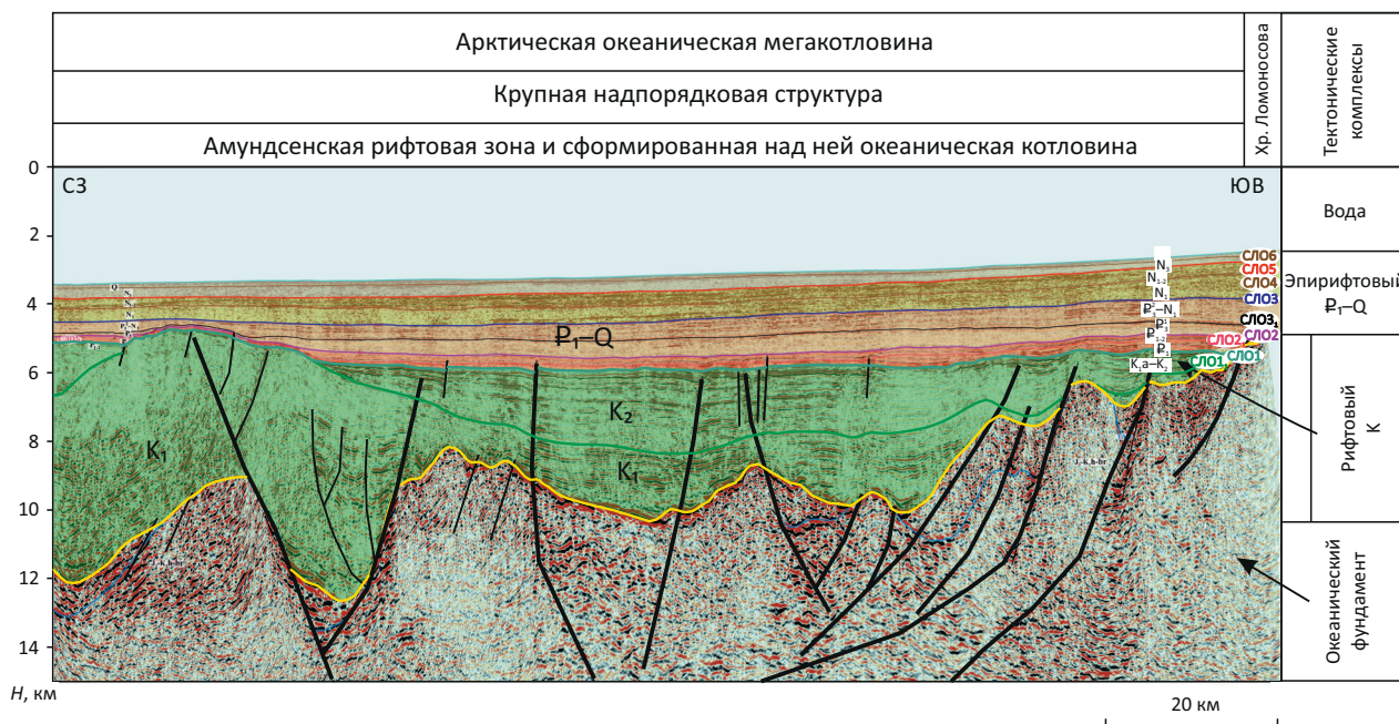
Рис. 7. Строение Амундсенской рифтовой зоны и сформированной над ней океанической котловины (сейсмическая основа ОАО «МАГЭ», 2014)
