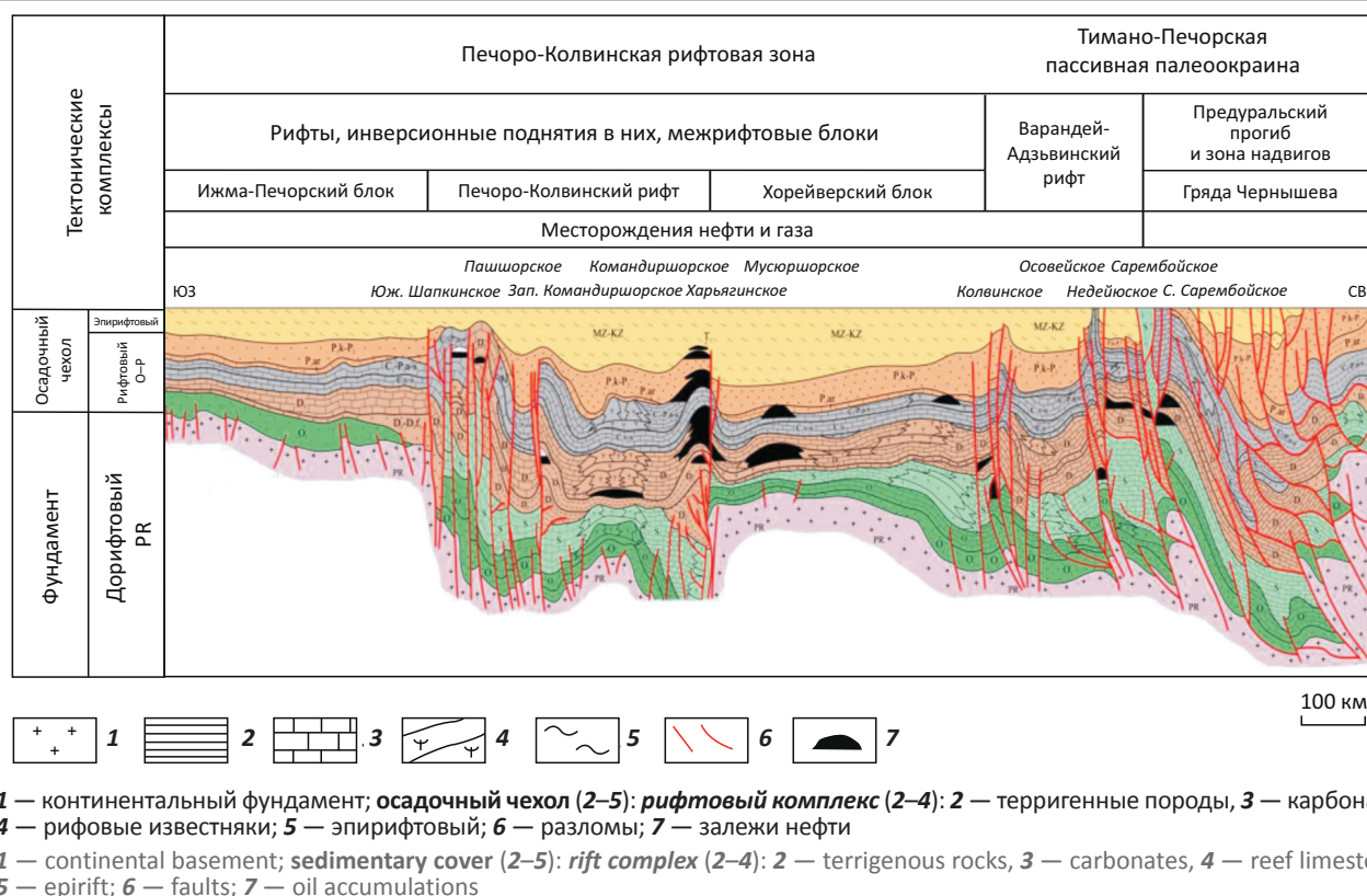
Рис. 9. Строение Печоро-Колвинской рифтовой зоны и Тимано-Печорской пассивной континентальной палеоокраины Fig. 9. Architecture of Pechora-Kolvinsky rift zone and Timan-Pechora passive continental paleo-margin
