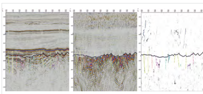
Рис. 6 — Разрезы кубов сейсмических данных (слева направо): куб зеркальной компоненты, куб рассеянной компоненты, куб Anttracking-a. Fig. 6. — Sections of seismic data cubes (from left to right): mirror component cube, diffuse component cube, Anttracking cube.
