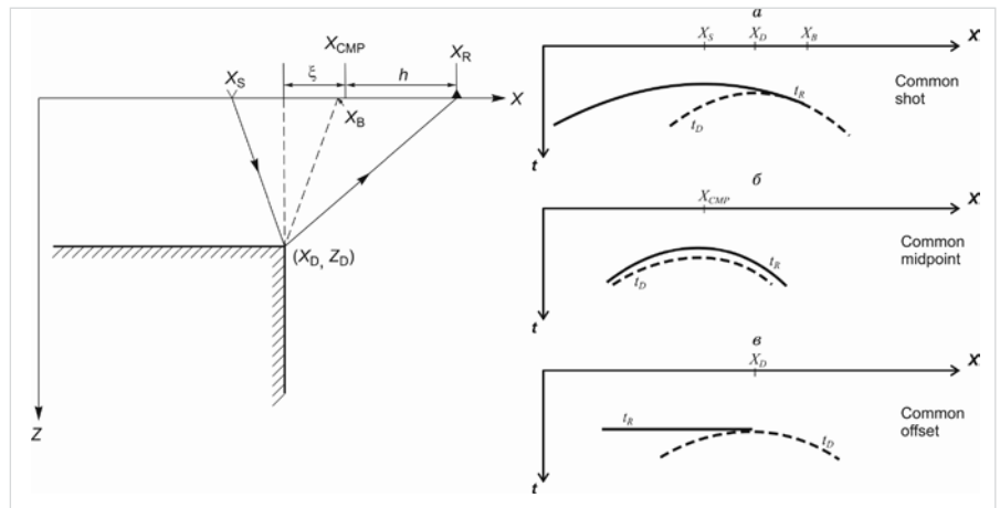
Рис. 2 — Годографы отраженной и дифрагированной волны в различных системах наблюдений для модели прямоугольного клина [4]. Fig. 2. — Hodographs of the reflected and diffracted waves in various observation systems for the rectangular wedge model [4].
