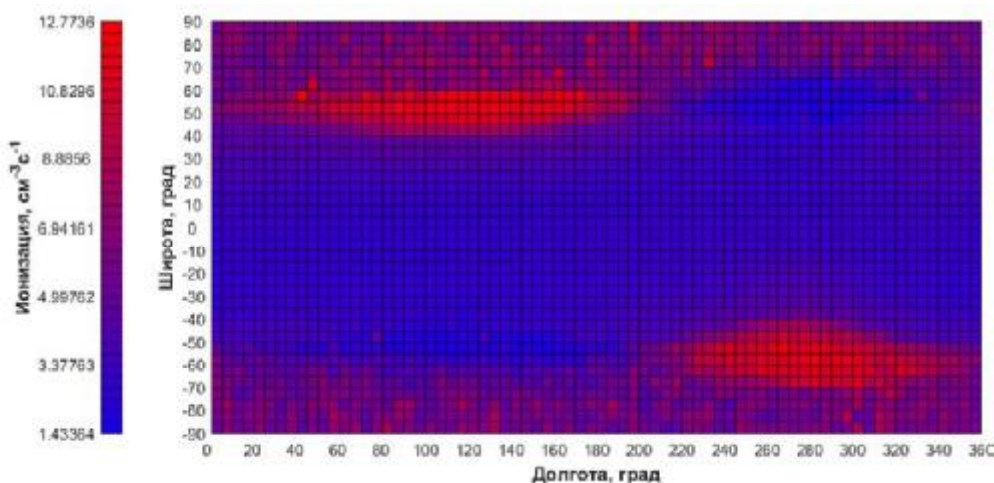
Рис. 1. Типовая ионограмма, позволяющая производить оценку скорости ионизации всей атмосферы Земли на высоте 5 км, полученная путем моделирования прохождения протонов первичных ГКЛ во время минимума солнечной активности. Данные для высот от 1 км до 80 км, с шагом в 1 км можно найти на сайте проекта [http://ruscosmics.ru]
