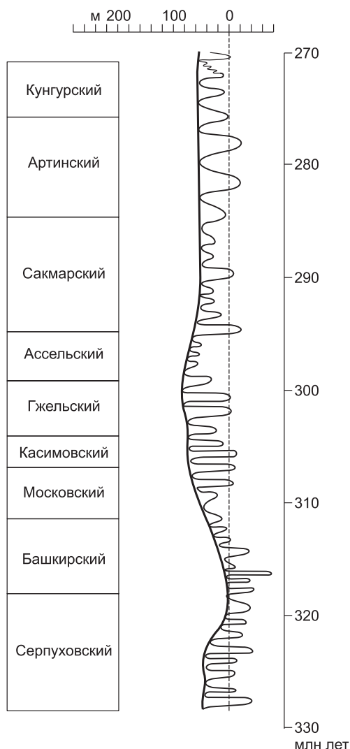
Рис. 1. Флуктуации уровня океана, предполагаемые с серпуховского века раннего карбона до кунгурского века ранней перми, по [Naq, Schutter, 2008] с изменениями.
