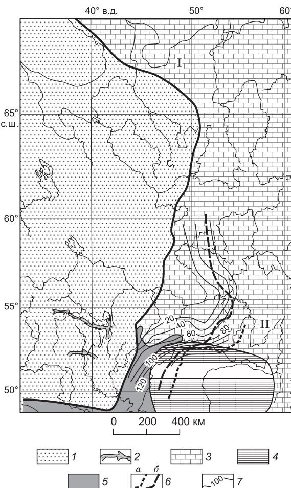
Рис. 2. Восточно-Европейская платформа в башкирском веке, по [Геология..., 1967] с изменениями.
