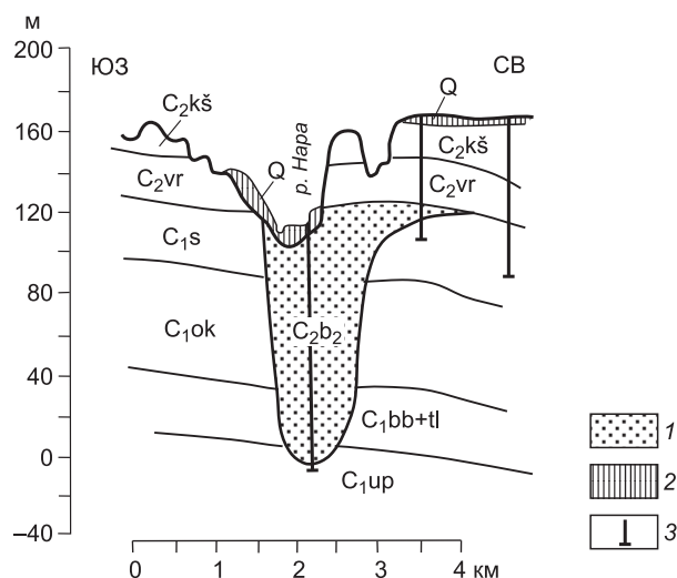
Рис. 9. Профиль Азовской палеодолины пред-позднебашкирского возраста в отложениях нижнего карбона на юге московской синеклизы в районе г. Серпухов, по [Махлина и др., 2001a] с изменениями.
