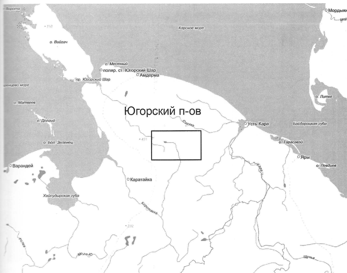
Рис. 1. Местоположение района работ Fig. 1. Location of the study area
