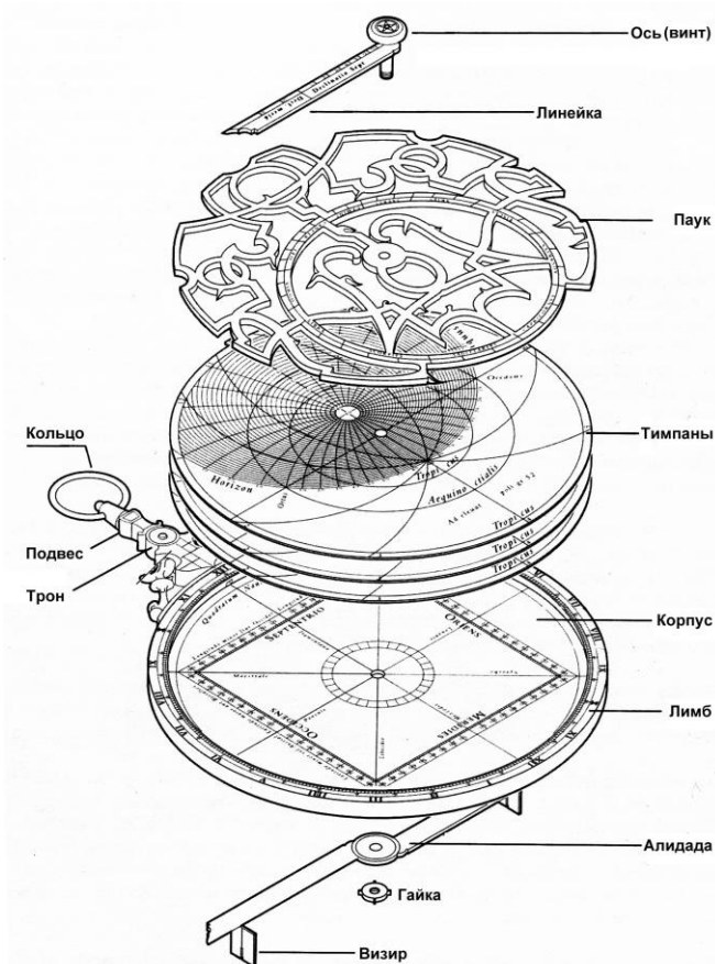
Рисунок 1 – основные детали западной астрлябии
