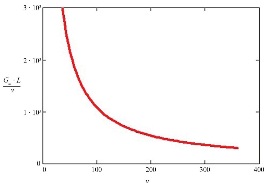
Рис. 1. Импульс вертикальной силы H \cdot s , действующей со стороны автомобиля на дорожное покрытие, в зависимости от скорости движения автомобиля, км/ч, с учетом только его силы тяжести ( L = 3 м — база автомобиля, G_m = 10 кН)
