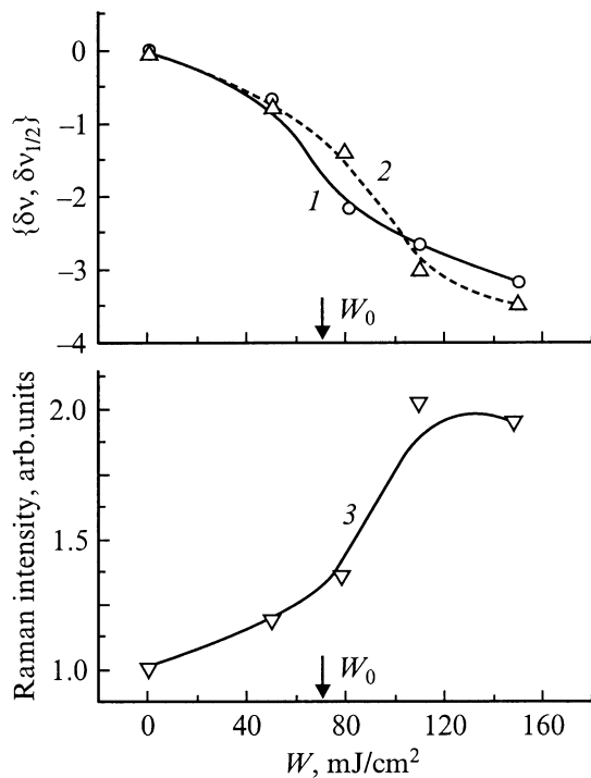
Рис. 4. Изменение параметров КР света от реальных поверхностей германия, подвергнутых предварительному воздействию импульсного лазерного луча с плотностью падающей энергии в центре пятна W : 1 — частотный сдвиг рамановской линии \delta\nu , 2 — уменьшение ширины линии на полувысоте \delta\nu_{1/2} , 3 — рост интенсивности комбинационного рассеяния.
