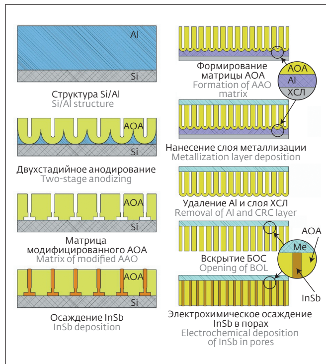
Рис.3. Схематическое изображение последовательности технологических процессов формирования InSb нанопроводов в матрицах AAO на n-Si подложках (a) и в порах нанопористых подложек из AAO (b) Fig.3. Schematic representation of sequence of processing for formation of InSb nanowires in AAO matrixes on n-Si substrates (a) and in pores of nanoporous AAO substrates (b)
