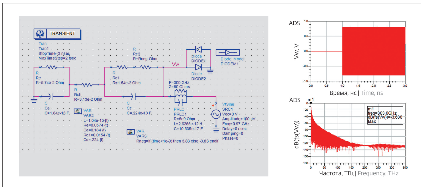
Рис.12. Генерация на частоте 303,0 ГГц
