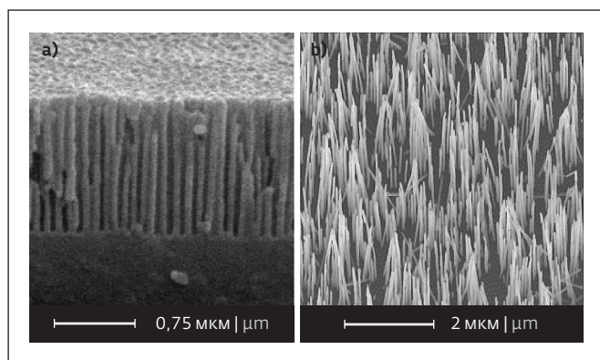
Рис.4. Электронно-микроскопические снимки матриц АОА на кремниевой подложке для формирования матрицы нанопроводов (а) и массива нанопроводов InSb на подложке после селективного удаления матрицы АОА (б)
