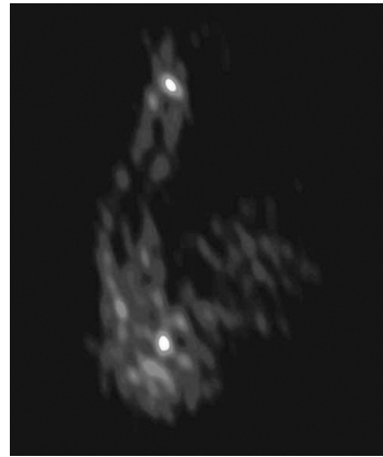
Карта радиоисточника 3С84 в активной эллиптической галактике NGC 1275 в скоплении галактик созвездия Персея. По данным наземно-космического интерферометра “Радиоастрон”. ФИАН.
